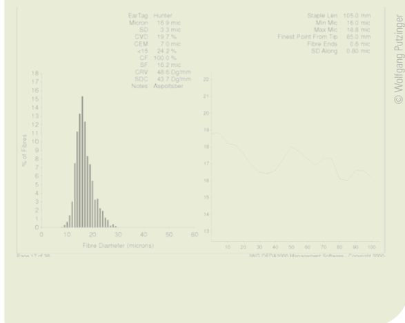
Abbildung 39 Faserdiagramm aus dem Labor
